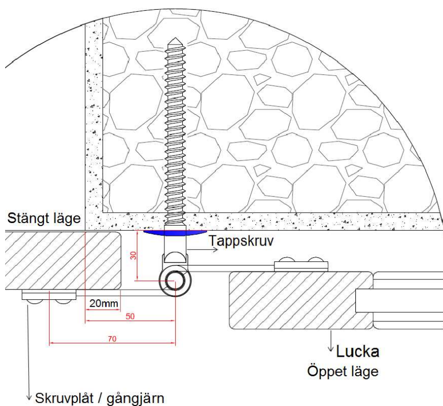
Detalj montering
